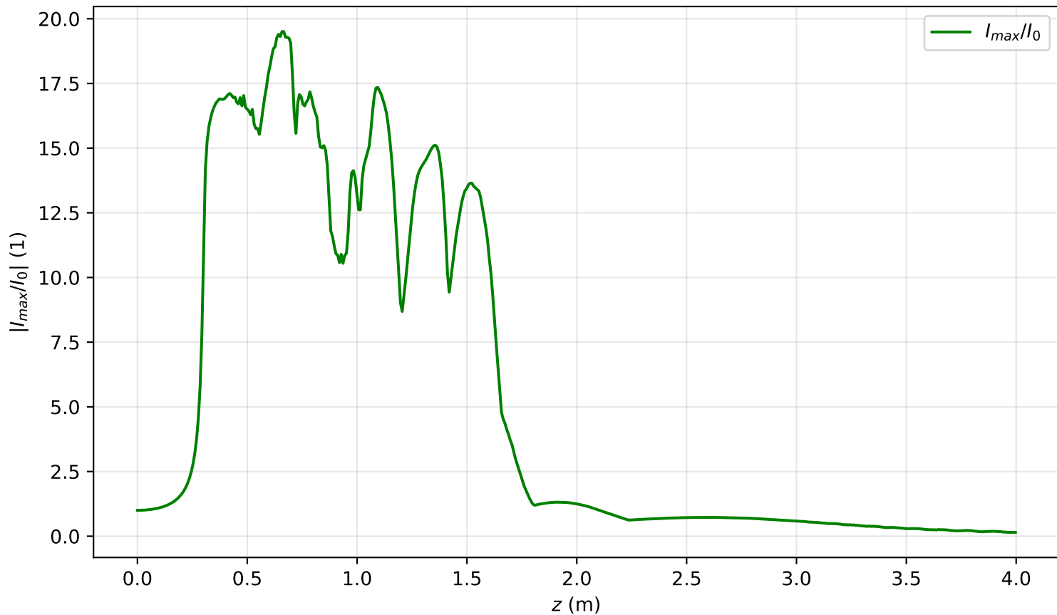
I_{\max}(r=0, z)/I_0 , Pin=9.2Pcr
